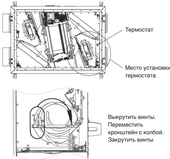
Рис. 3 Схема изменения положения термостата Alpha 400 Compact, Alpha 550 Compact
