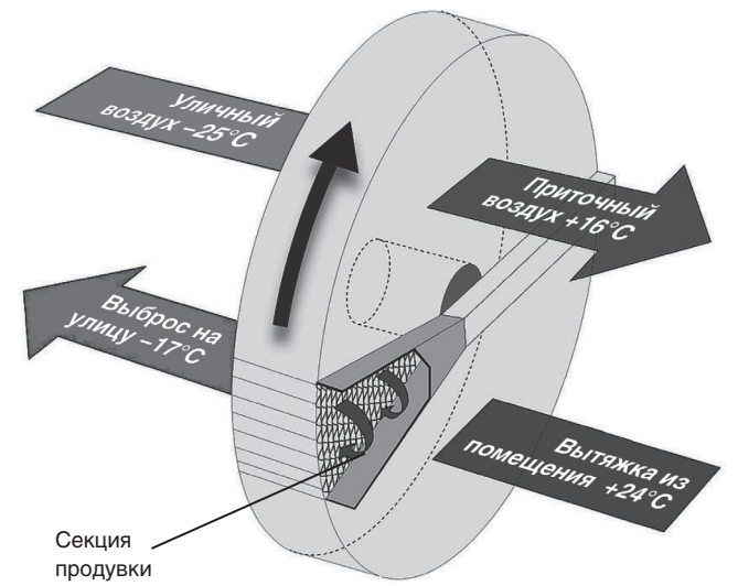
Рис. 6 Принцип работы роторного рекуператора
