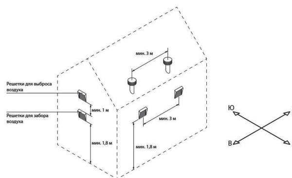
Рис. 5 Монтаж уличных решеток и клапанов
