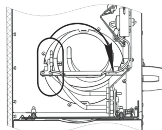
Рис. 3 Схема изменения положения термостата Alpha 400 Compact, Alpha 550 Compact
