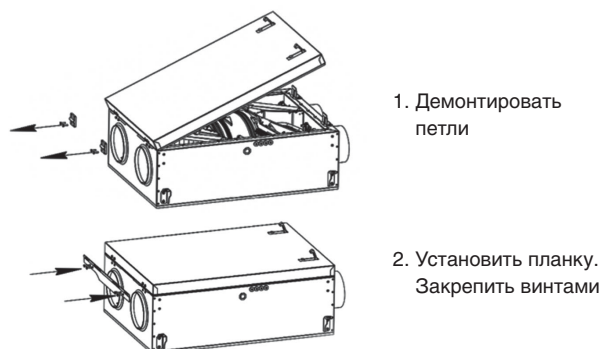
Рис. 4 Съемные петли Alpha 400 Compact, Alpha 550 Compact
