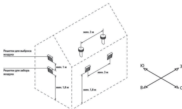
Рис. 5 Монтаж уличный решеток и клапанов
