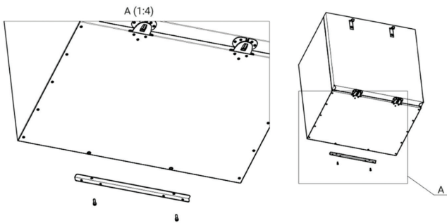
Рис. 3 Нижняя монтажная планка
