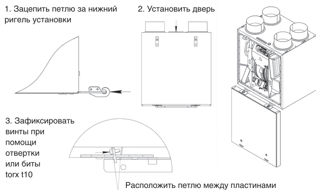
Рис. 4 Крепление двери на откидных петлях
