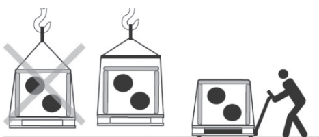
Рис. 1А Подъем и перемещение вентустановок
