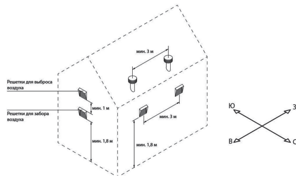
Рис. 5 Монтаж уличных решеток и клапанов
