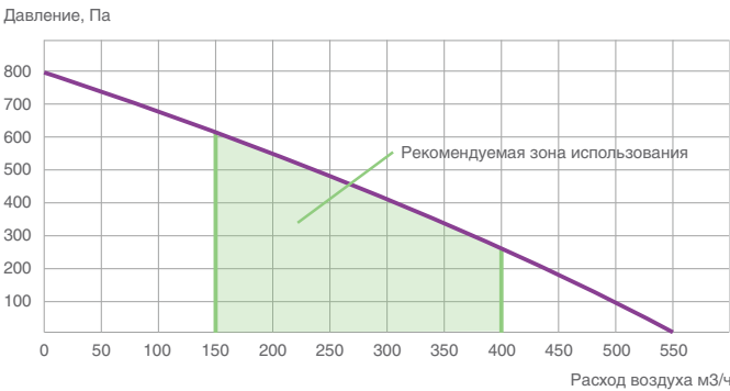
График статического давления
