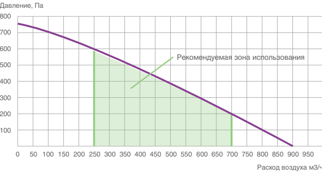
График статического давления
