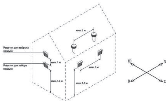
Рис. 5 Монтаж уличный решеток и клапанов
