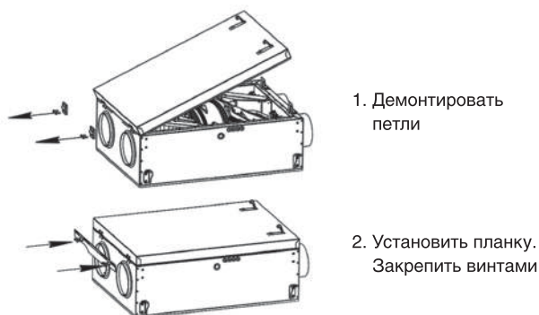
Рис. 4 Съемные петли на примере Alpha 400 compact
