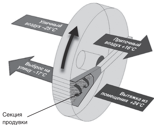
Рис. 6 Принцип работы роторного рекуператора
