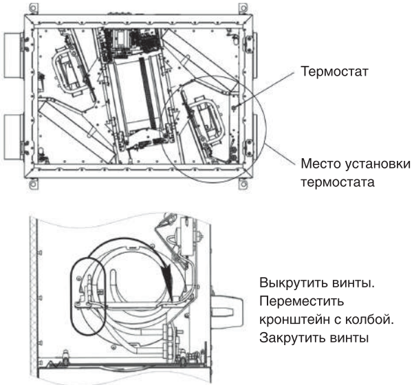
Рис. 3 Схема изменения положения термостата на примере Alpha 400 Compact
