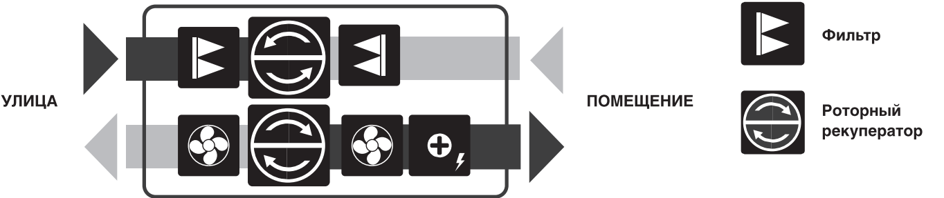
Функциональная схема установок Alpha 550 Compact, Alpha 700 Compact
